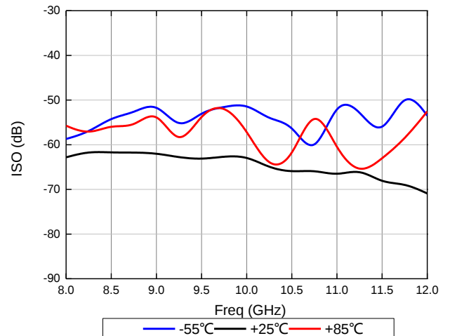
隔离度 (CW)
