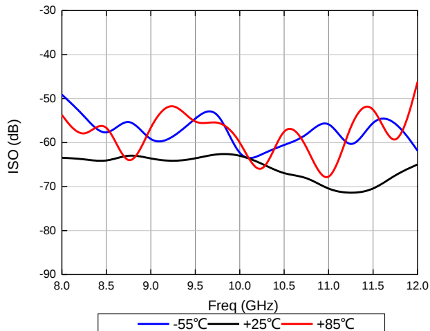
隔离度 (Pulse)
