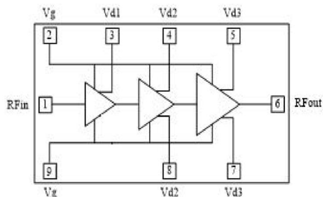
YGPA128-0812C1 功能框图
