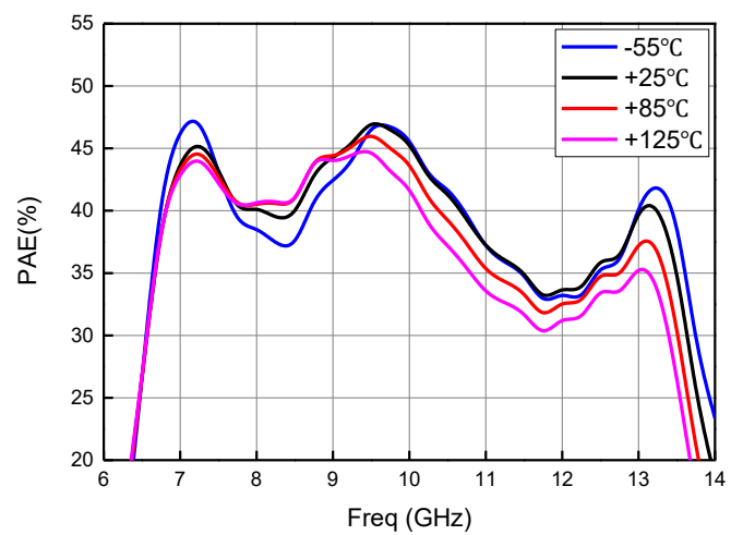
功率附加效率 (Pulse)
