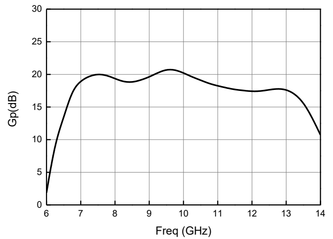
功率增益 (CW)
