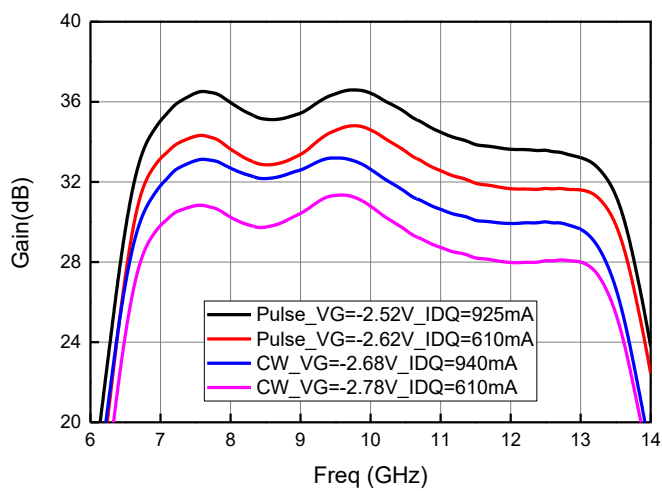
小信号增益
