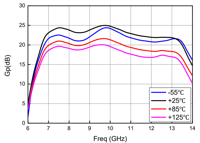
功率增益 (Pulse)
