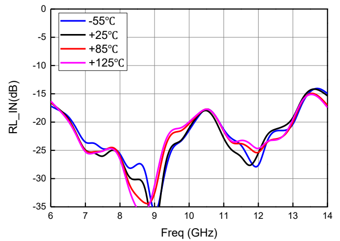
输入回波损耗 (Pulse)
