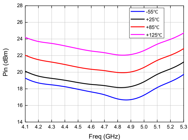
输入功率@OP7dB
