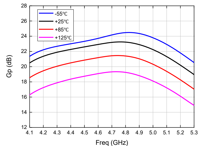
功率增益@OP7dB
