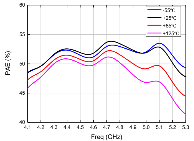
功率附加效率@OP7dB
