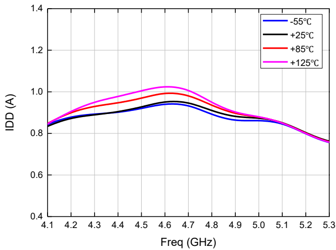
动态电流@OP7dB
