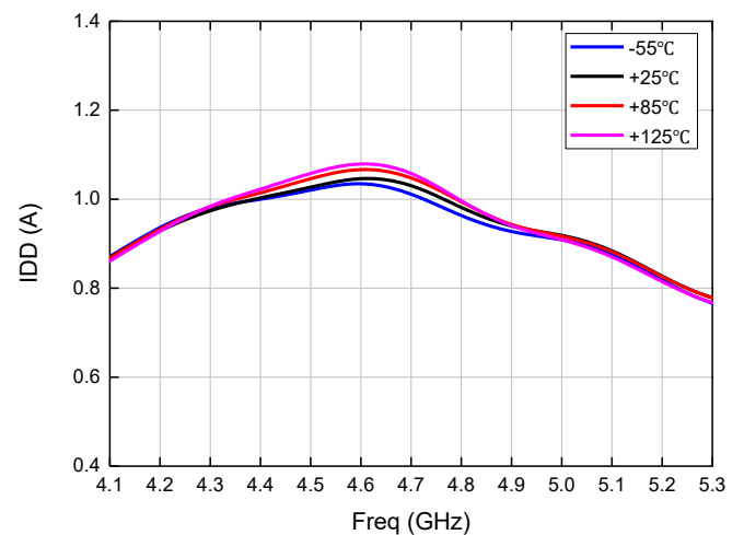
饱和动态电流
