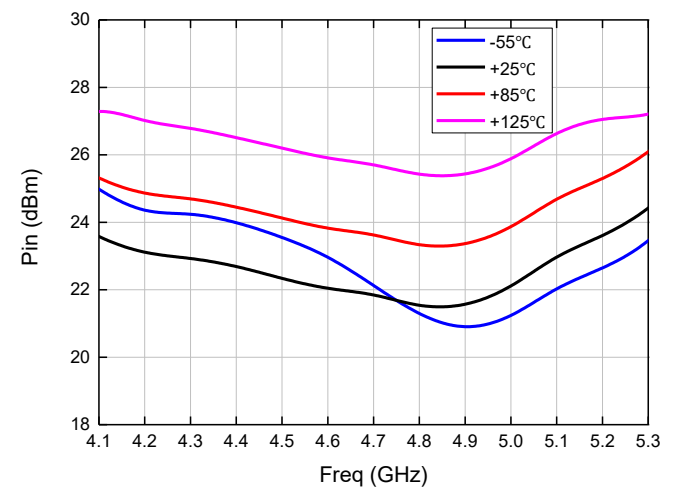
饱和输入功率
