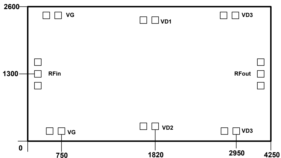
芯片端口图 (单位: \mu\text{m} )
