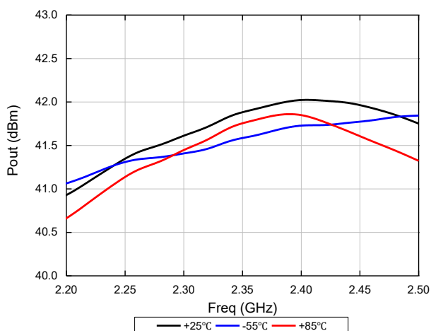
输出功率@P5dB
