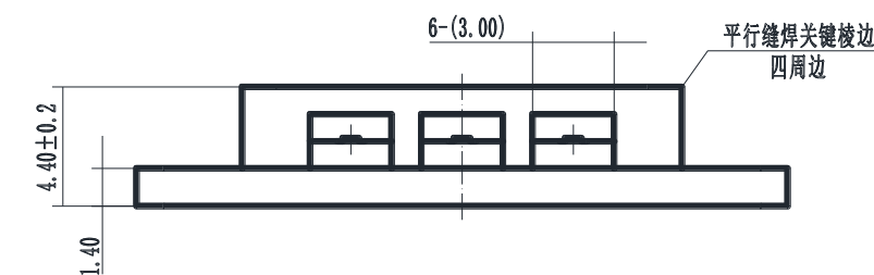
外形尺寸 (单位: mm)
