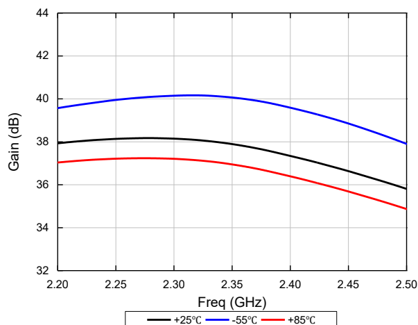
小信号增益
