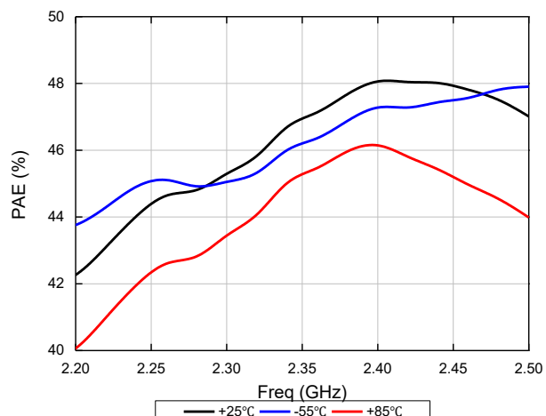
功率附加效率@P5dB
