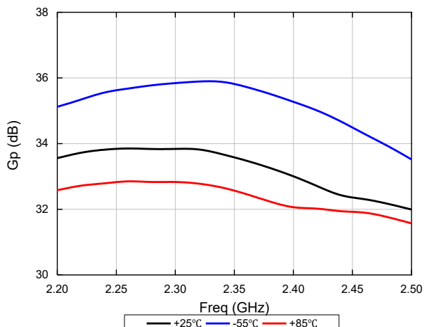
功率增益@P5dB
