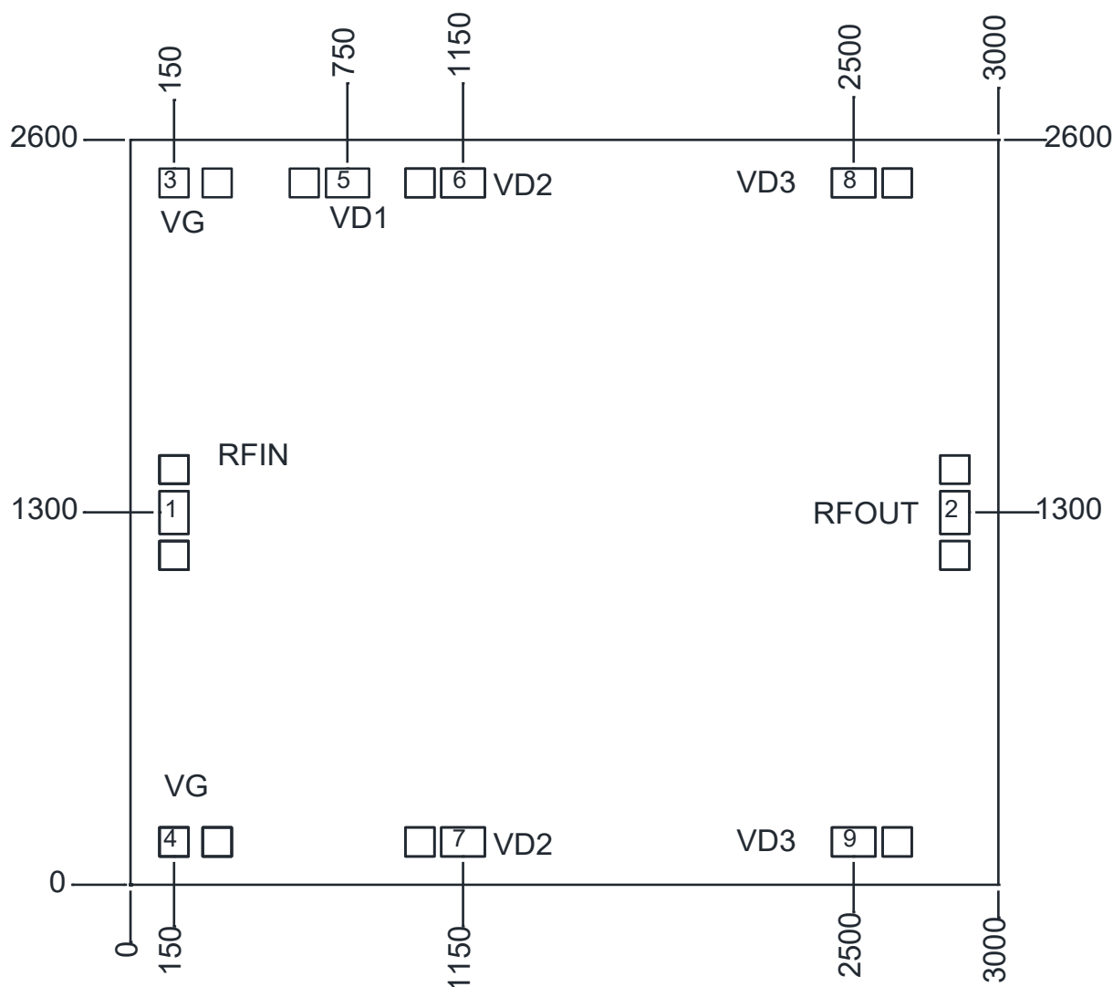
芯片端口图（单位：μm）
