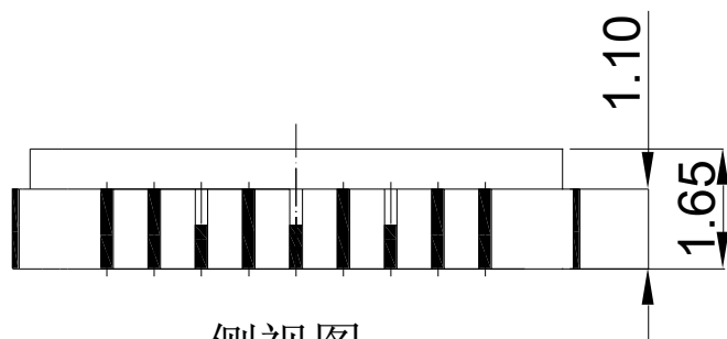
侧视图
