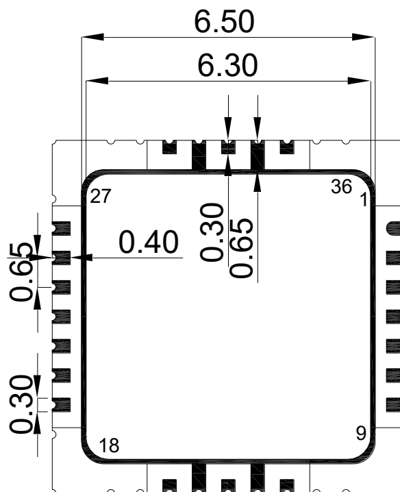
仰视图
