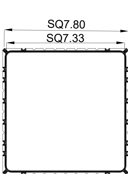
正视图
