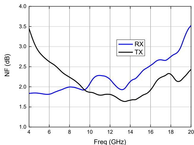
噪声系数
