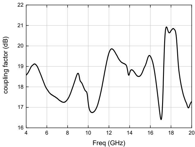
耦合系数
