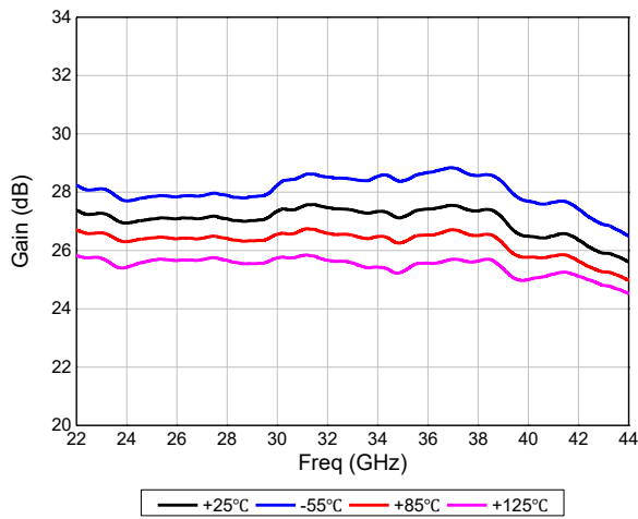
小信号增益
