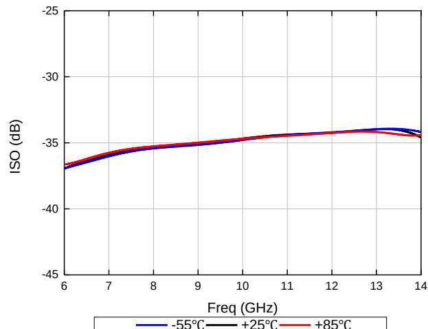
反向隔离度
