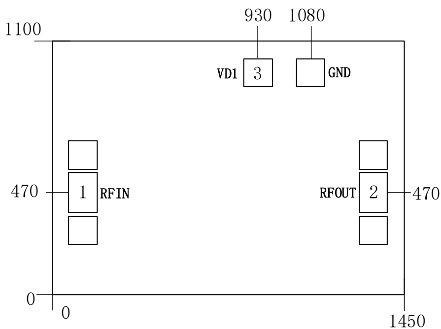
芯片端口图 (单位: \mu\text{m} )
