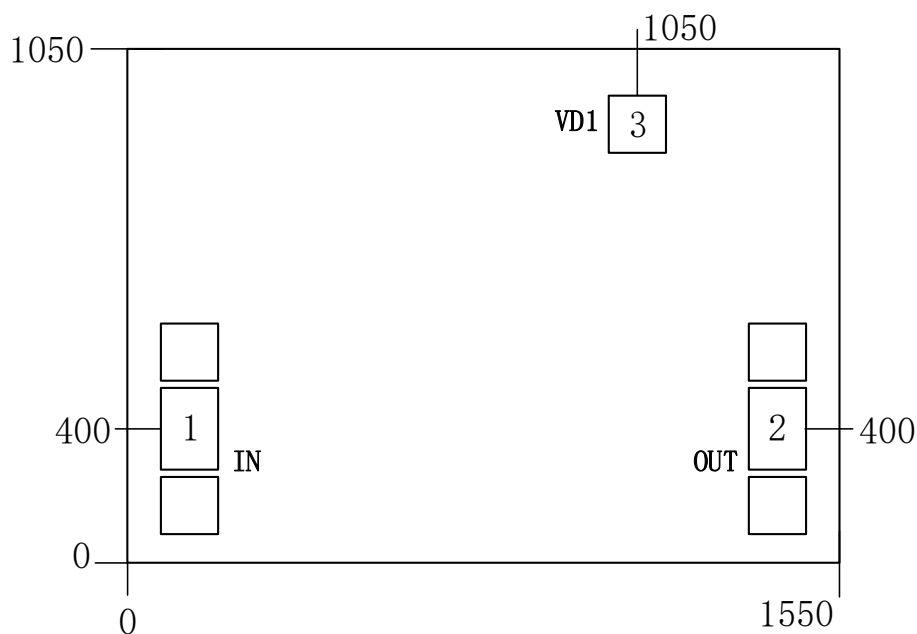
芯片端口图 (单位: \mu\text{m} )
