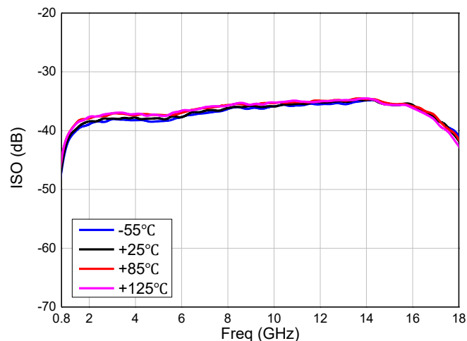
反向隔离度
