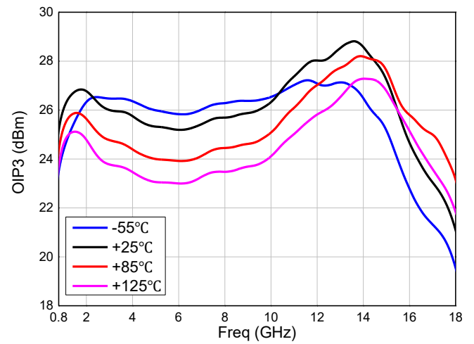
输出三阶交调功率@Pin=-20dBm
