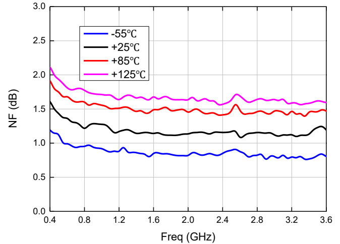
噪声系数
