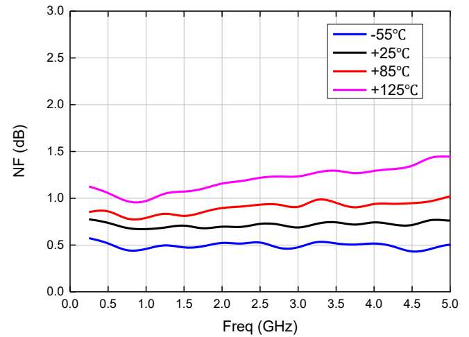
噪声系数
