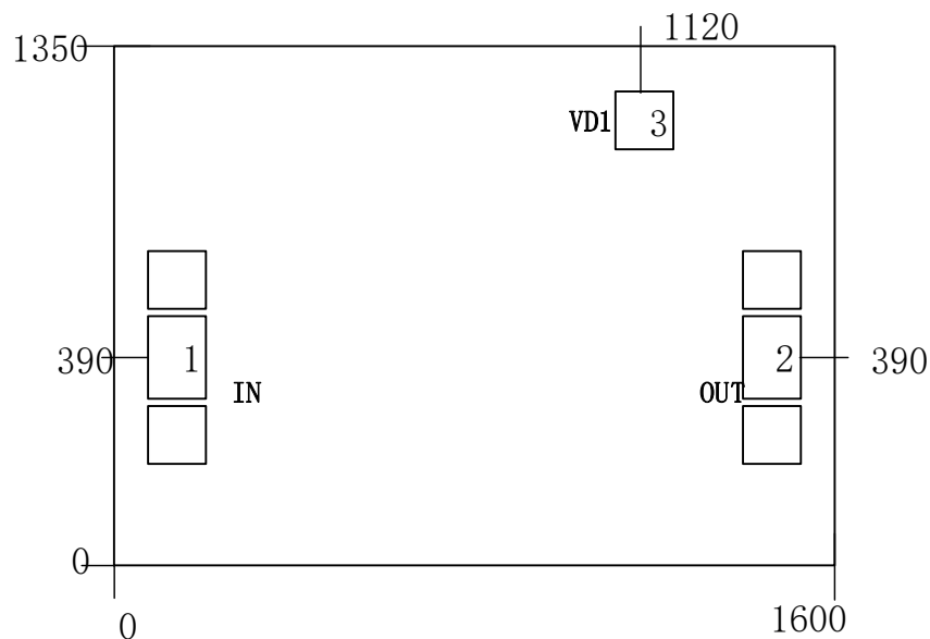
芯片端口图 (单位: \mu\text{m} )
