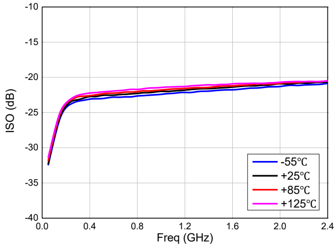
反向隔离度
