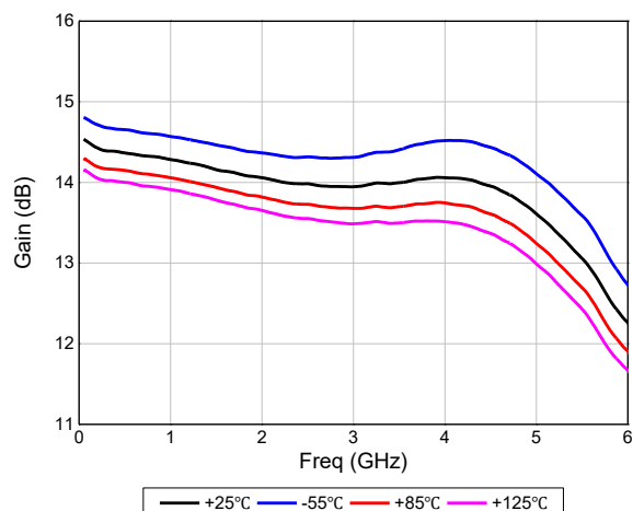
小信号增益
