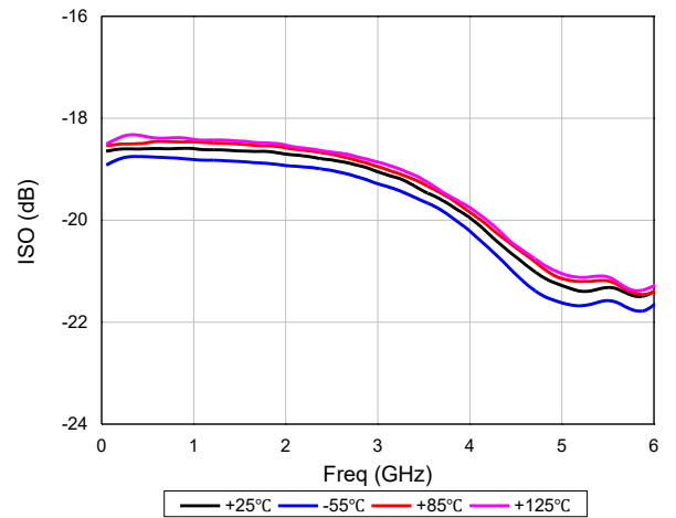
隔离度
