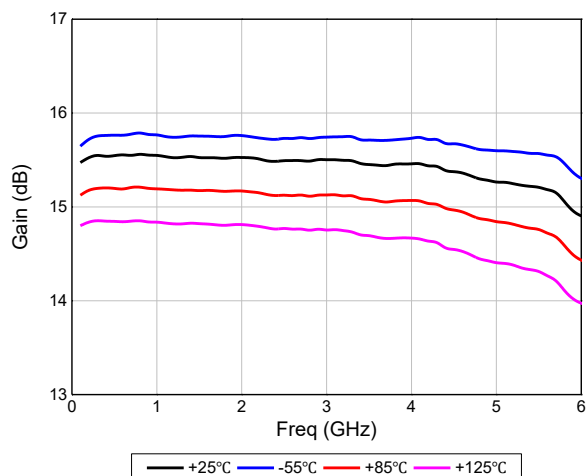
小信号增益
