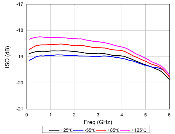
隔离度
