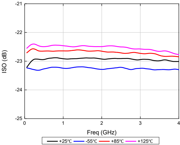
隔离度
