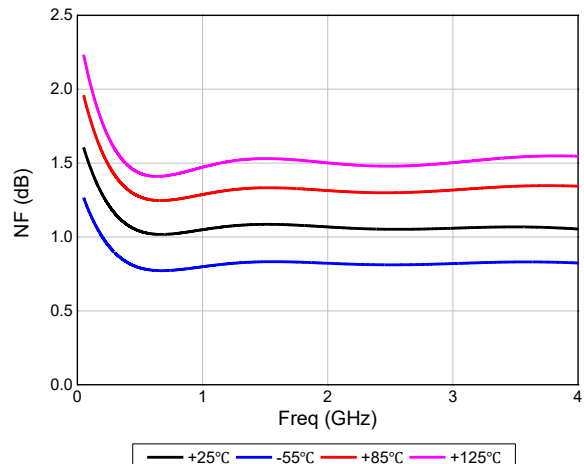
噪声系数
