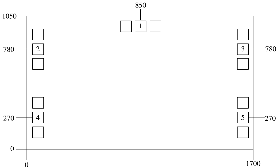
芯片端口图（单位：μm）
