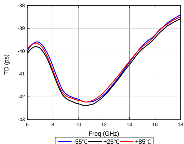
40ps 延时量
