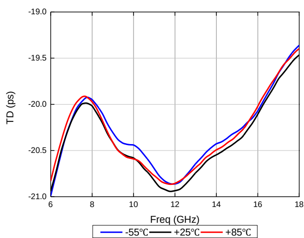
20ps 延时量
