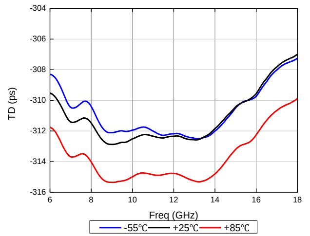
310ps 延时量
