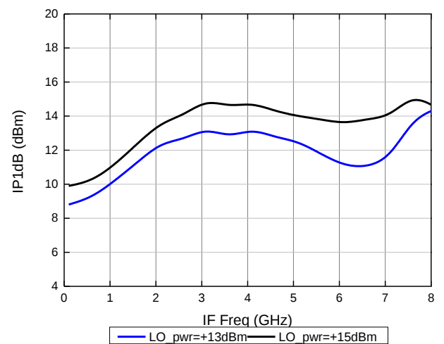
输入1dB压缩功率 (HLO=24GHz)
