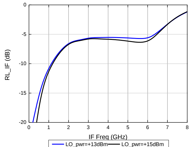
中频回波损耗 (HLO=24GHz)
