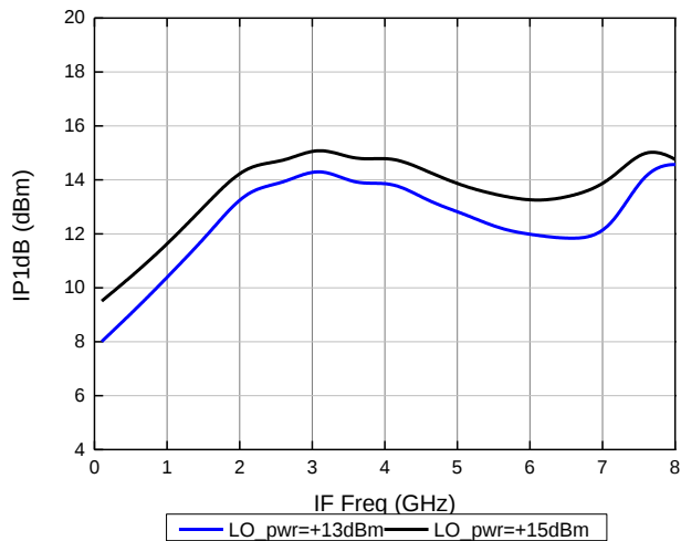
输入1dB压缩功率 (HLO=22GHz)
