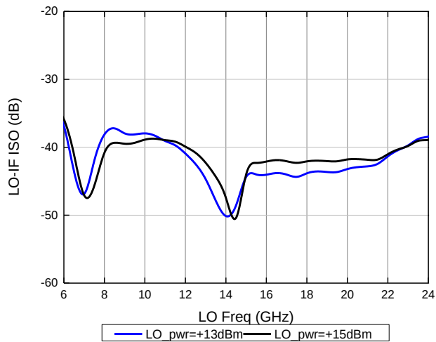
LO-IF隔离度
