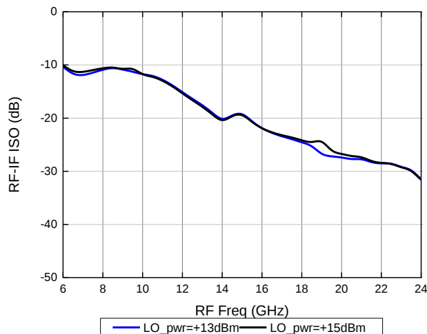
RF-IF隔离度
