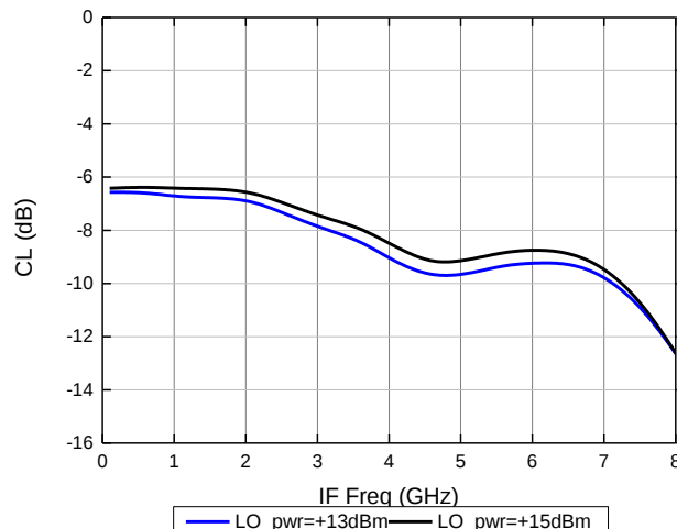
上变频损耗 (HLO=19GHz)
