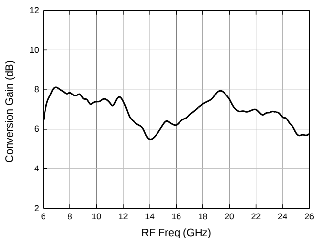
变频增益
