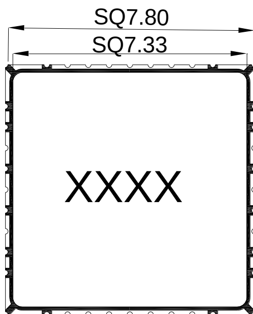
正视图
