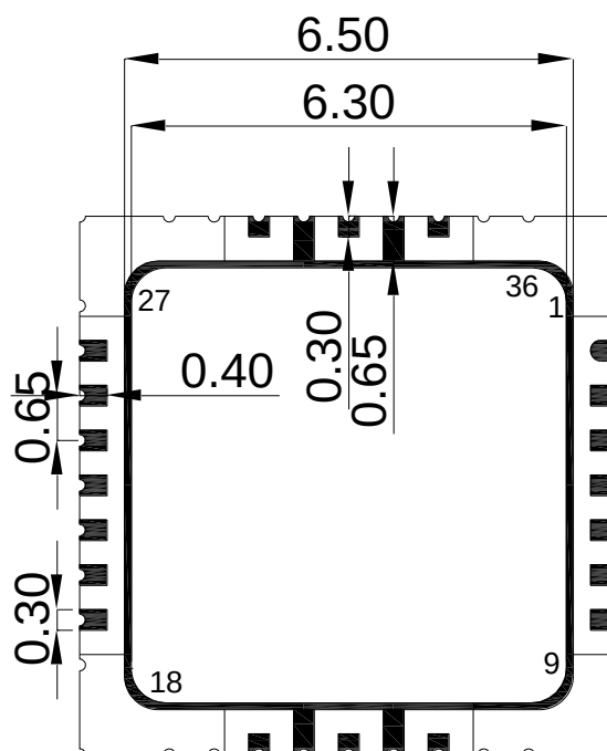
仰视图
