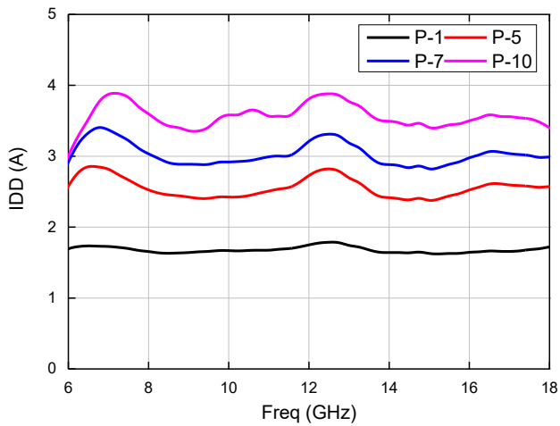
动态电流 (CW模式)
