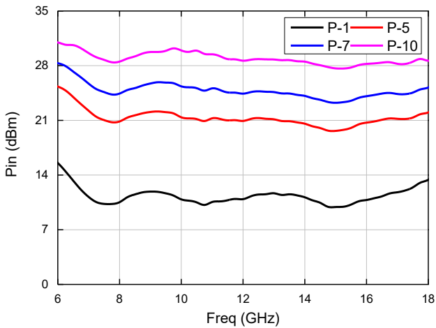
输入功率 (CW模式)
