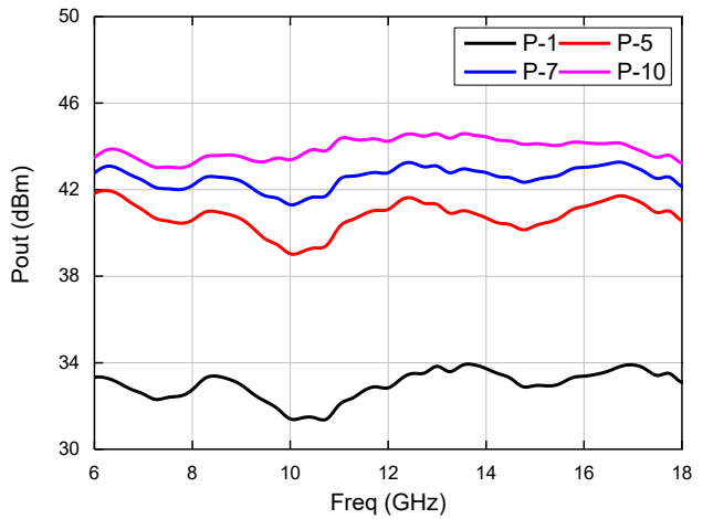
输出功率 (Pulse模式)
