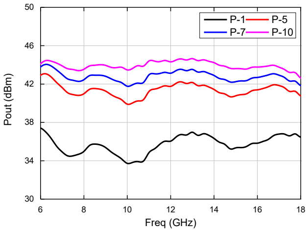
输出功率 (CW模式)
