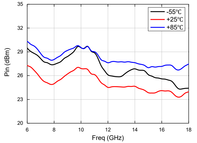
输入功率 (Pulse模式)
