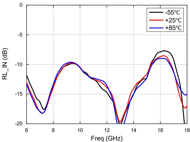
输入回波损耗（CW模式）
