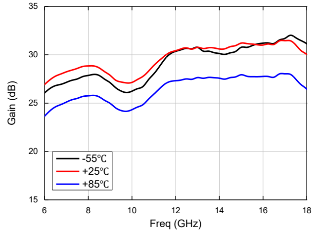
小信号增益（Pulse模式）
