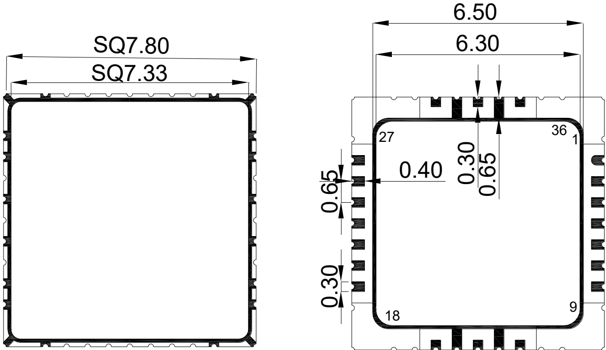
正视图
