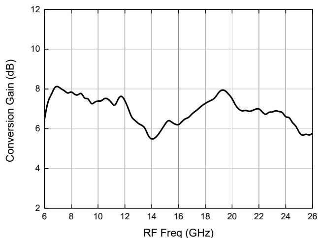
变频增益
