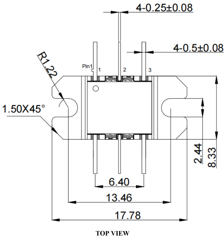
外形结构图 (单位: mm)
