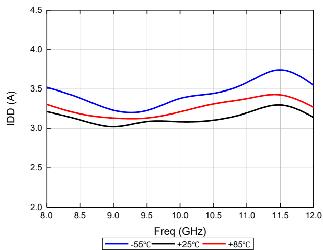
饱和动态电流 (Pulse)
