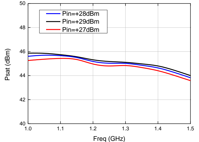
饱和输出功率@VD=+32V
