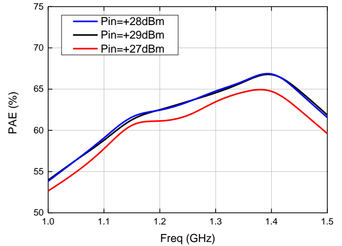
饱和功率附加效率@VD=+28V
