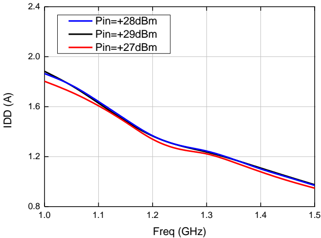
饱和动态电流@VD=+28V
