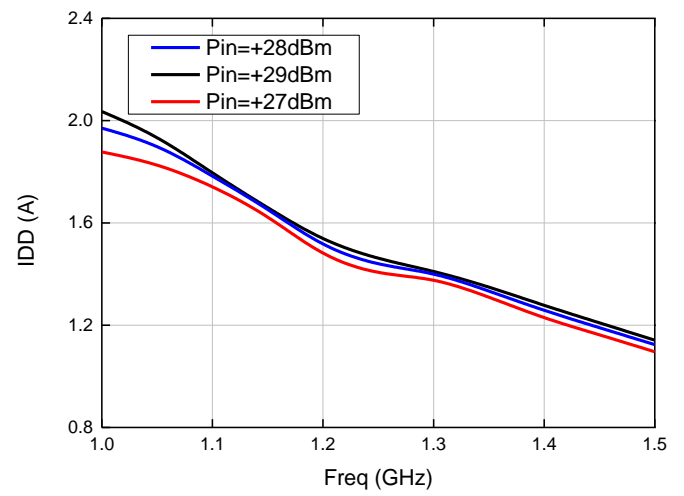
饱和动态电流@VD=+32V
