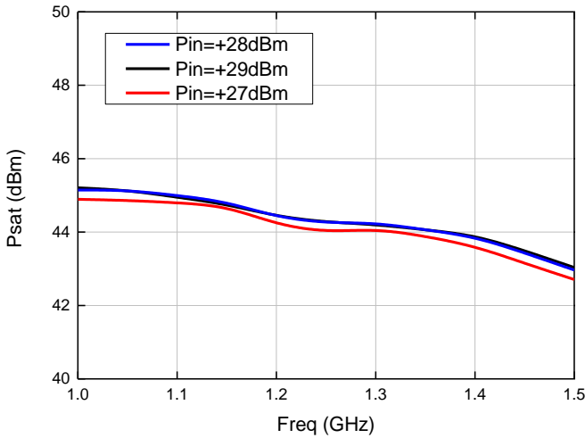
饱和输出功率@VD=+28V
