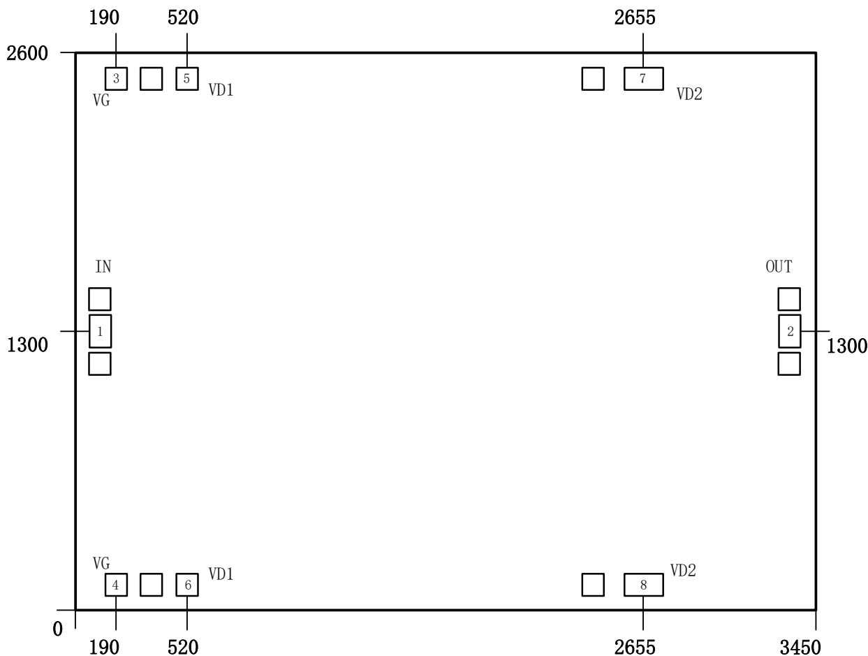
端口定义
