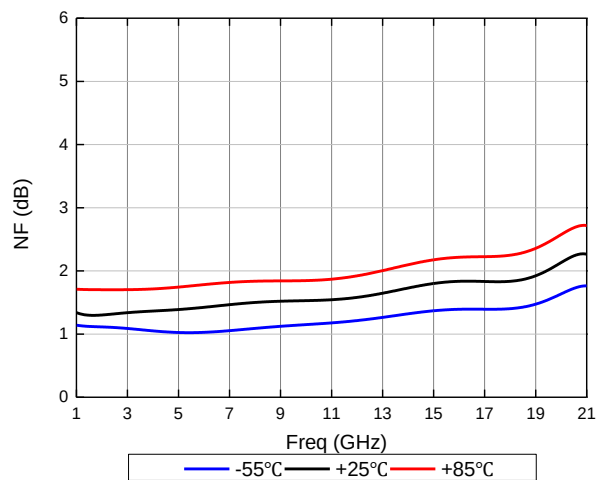
噪声系数
