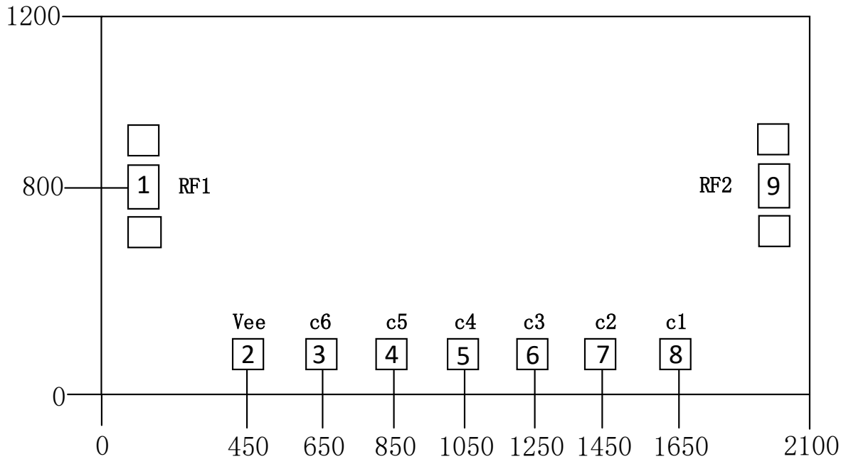
端口定义
