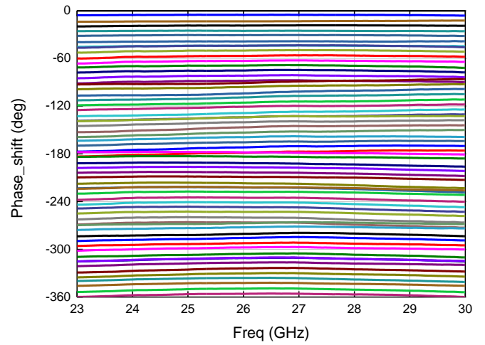
移相量
