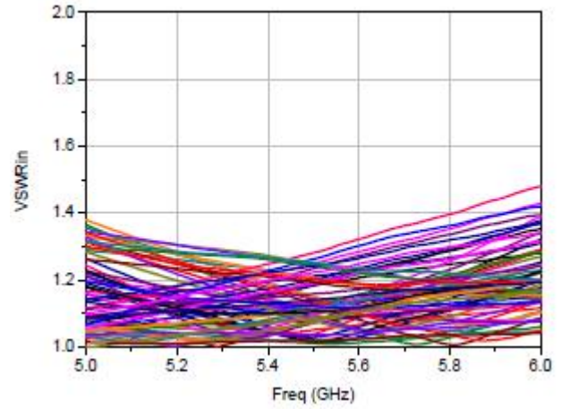
输入驻波
