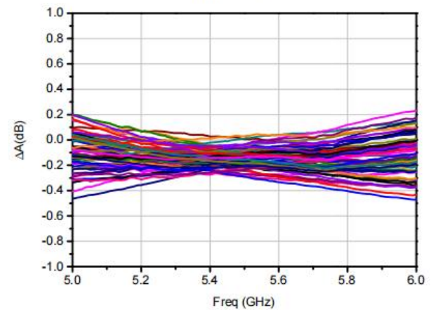
幅度波动
