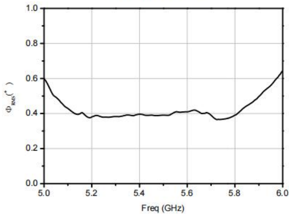
移相精度均方根
