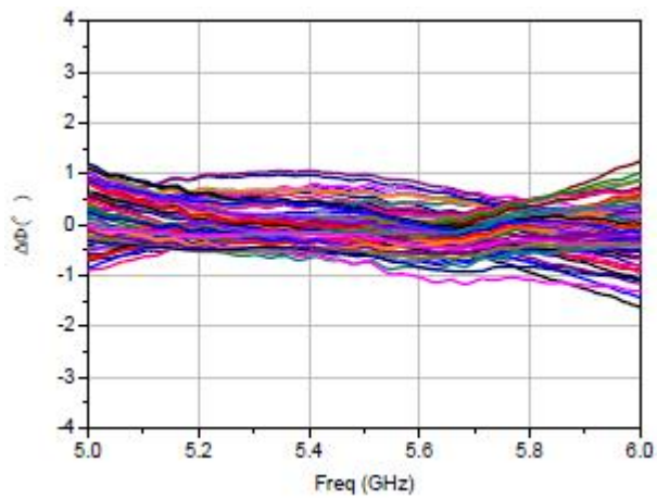
移相精度
