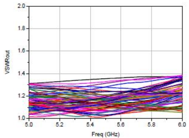
输出驻波
