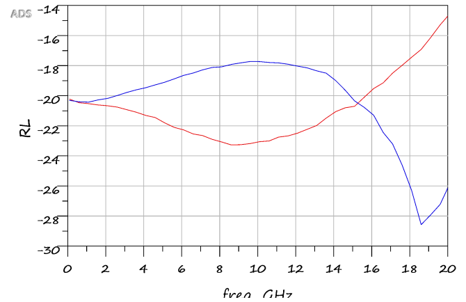
回波损耗
