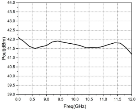
饱和输出功率 vs. 频率
