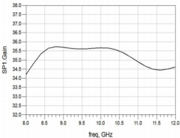
输入小信号增益 vs. 频率
