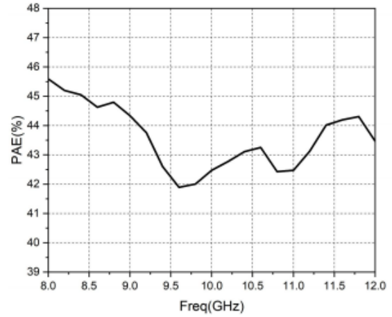
附加效率 vs. 频率
