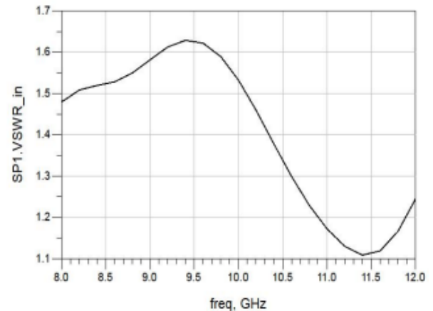
输入驻波 vs. 频率
