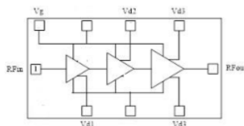
YGPA63-0812C1功能框图
