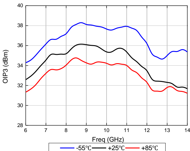
输出三阶交调@Pout=+7dBm
