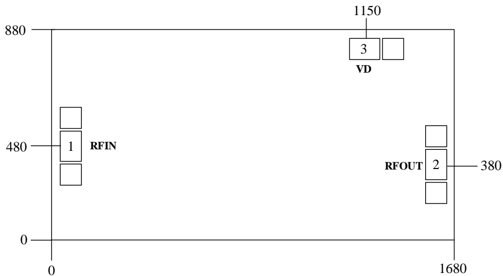
芯片端口图 (单位: \mu\text{m} )
